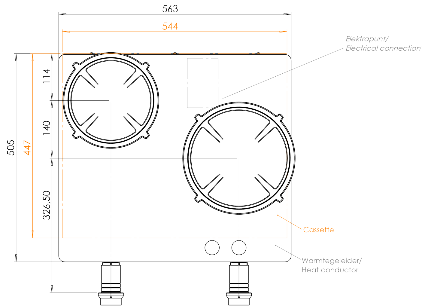
Bovenaanzicht / Top view
