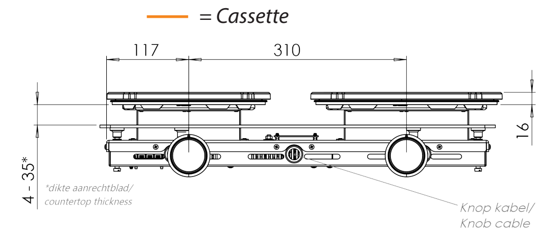
Vooraanzicht / Front view
